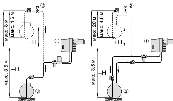
Однетрубная система
