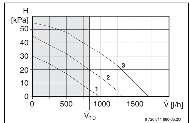
Рис. 30 Опалювальний насос
