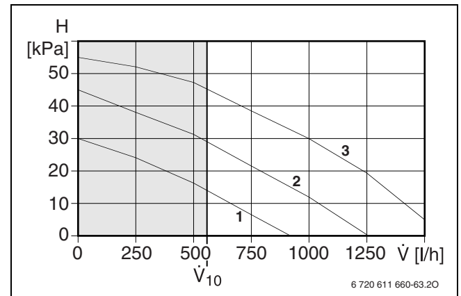
Рис. 28 Опалювальний насос
