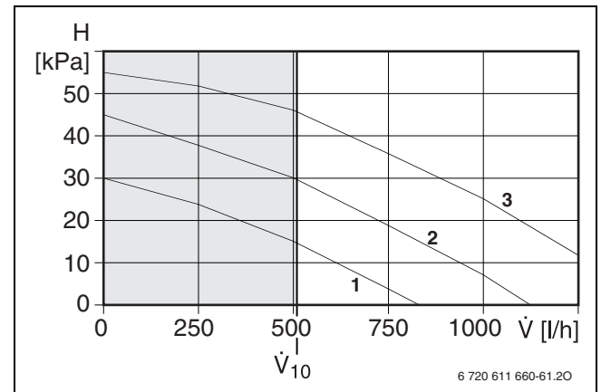
Рис. 26 Опалювальний насос
