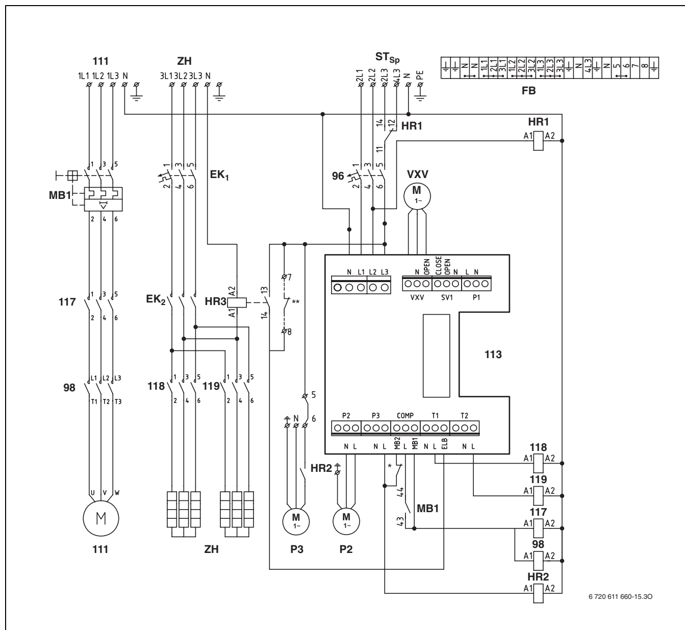
Рис. 11 Плата підключення
