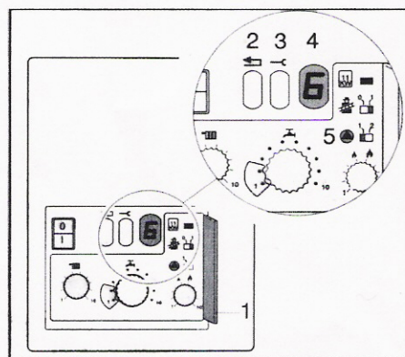
Рис. 2 Сервисное обслуживание, сигнализация режимов работы котла и неисправностей
