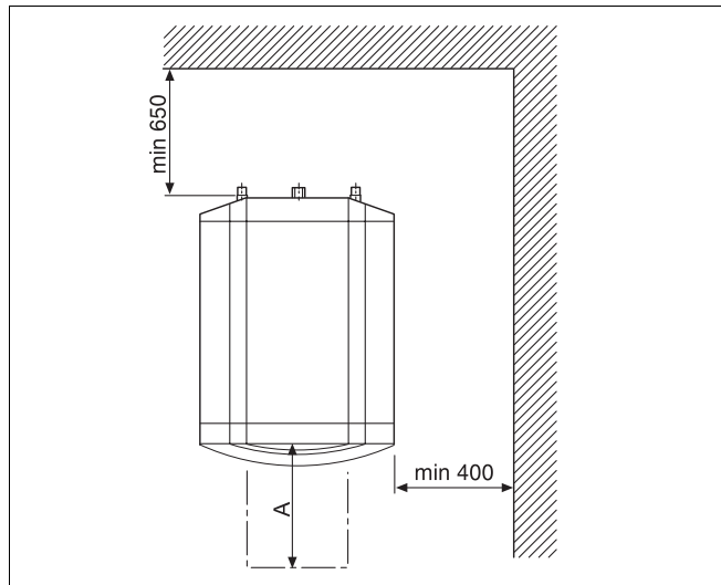
Рис. 8 Установка бака-водонагревателя (принципиальная схема)
