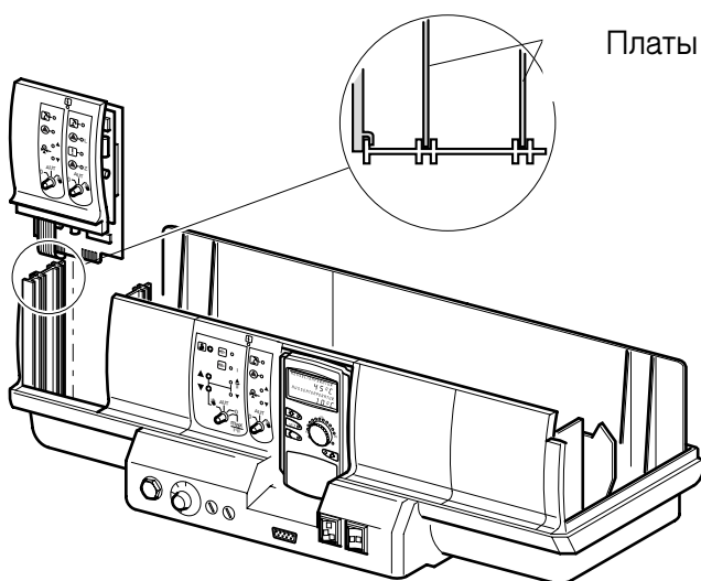
Рис. 4 Установка модуля
